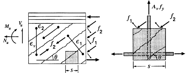
(d) Biaxial strains in web
